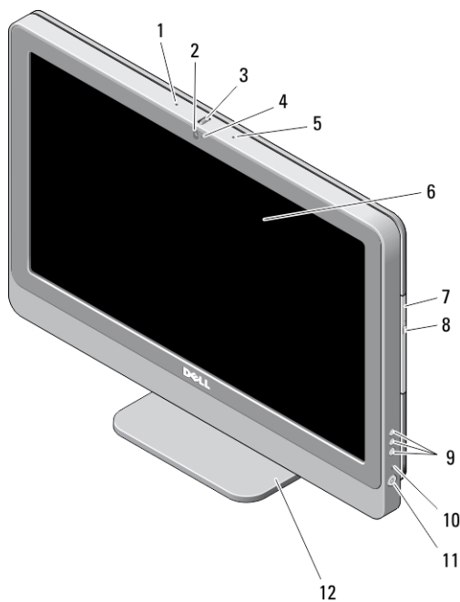
図 1. 正面図
